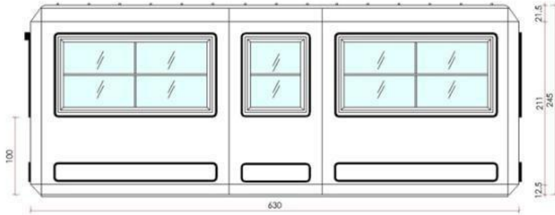
SAĞ YAN GÖRÜNÜŞ
